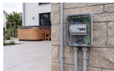
Beispielbild: eigener Stromkreis mit eigener Absicherung.
